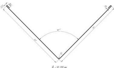
Конек плоский (уголок) с регулируемой шириной полки от 50 до 200мм
