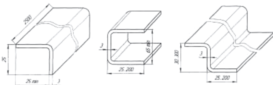
Профили, производимые на станке
