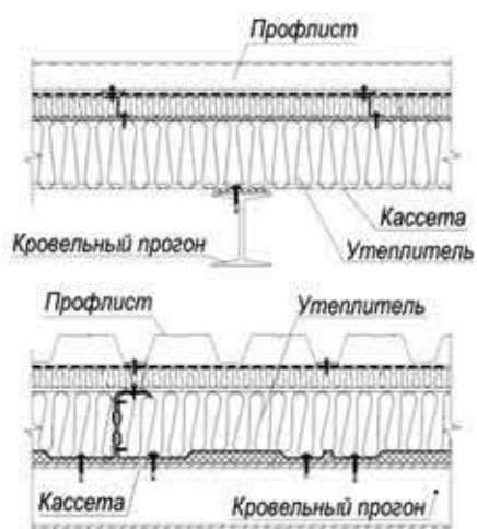
Конструкция кровли
